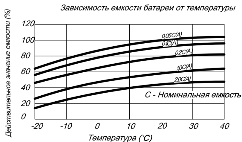
Рисунок 3 – Зависимость емкости батареи от температуры
