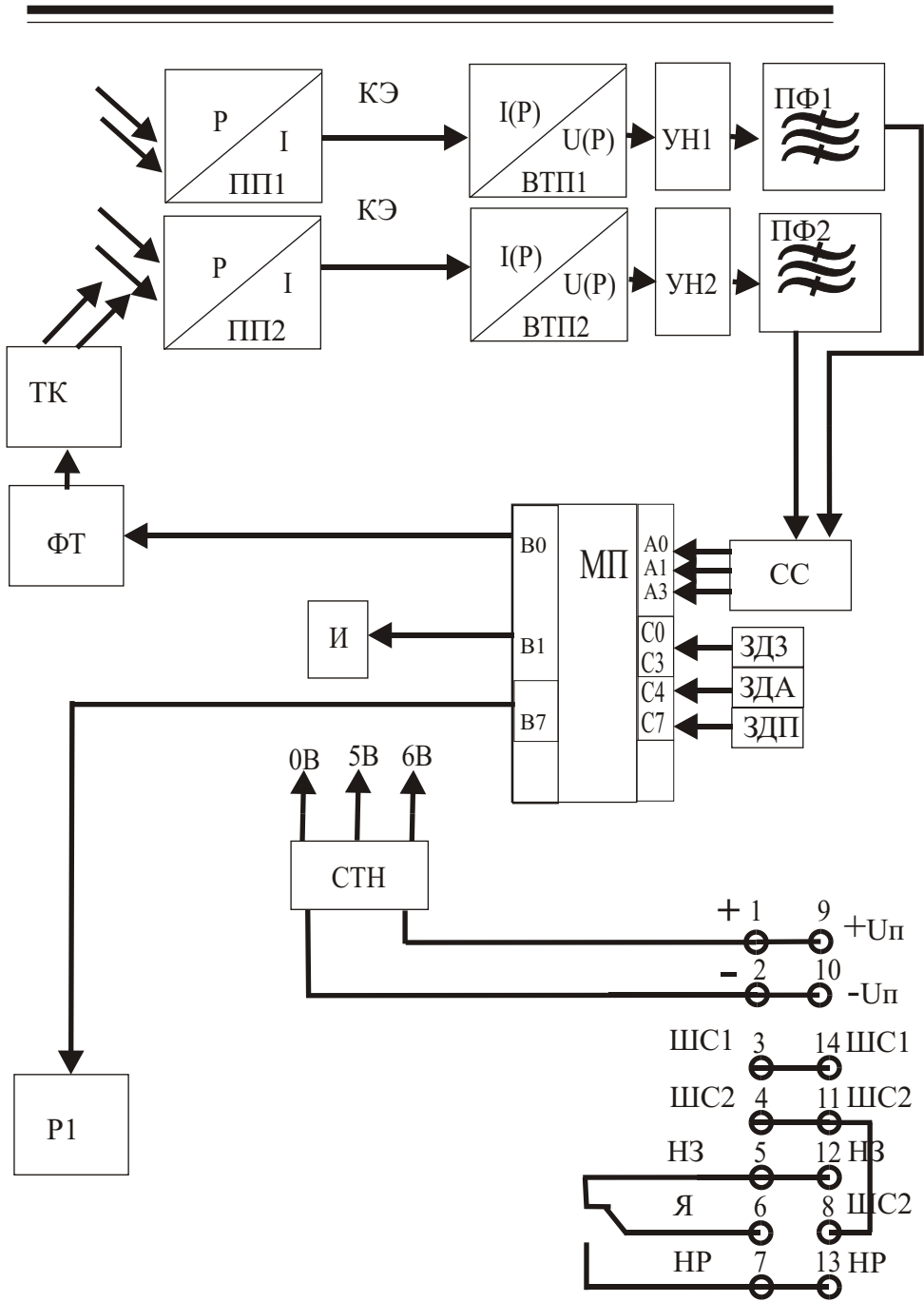
Рис3. Схема функциональная извещателя “Пульсар3-014СК”
