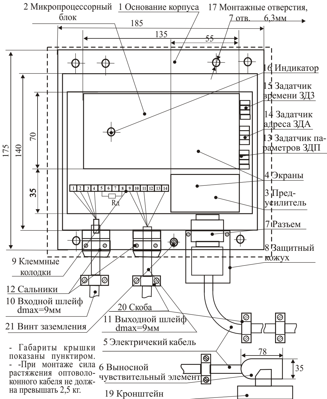
Рис 2 Извещатель пожарный пламени “Пульсар3-014” вид со снятыми крышкой и защитной пластиной
