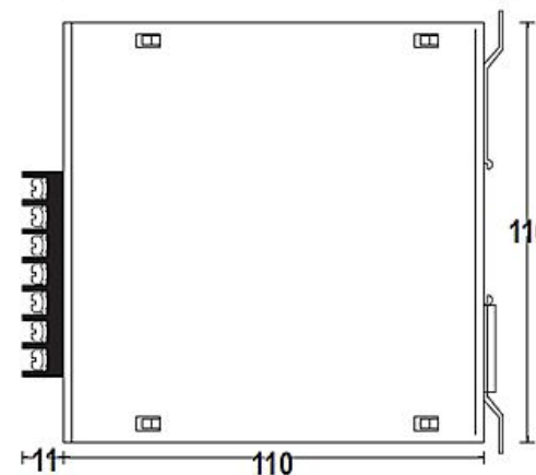
Габаритные размеры AD1500S и обозначения на передней панели
