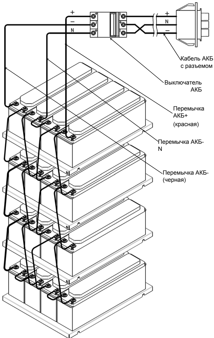
Рисунок 4 — Пример размещения и подключения аккумуляторных батарей в изделии
