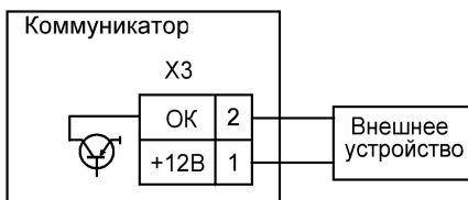
Рисунок 14.2 – Схема подключения внешнего устройства к коммуникатору
