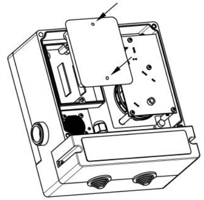
3. Вставить картридж и собрать в обратной последовательности.
