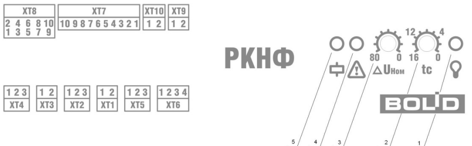
Рисунок 14. Лицевая панель РКНФ
