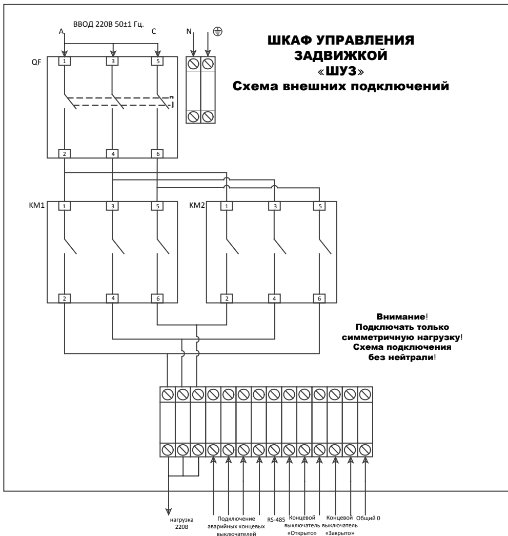
Рисунок 2-б. Схема внешних подключений к шкафу при 220В.
