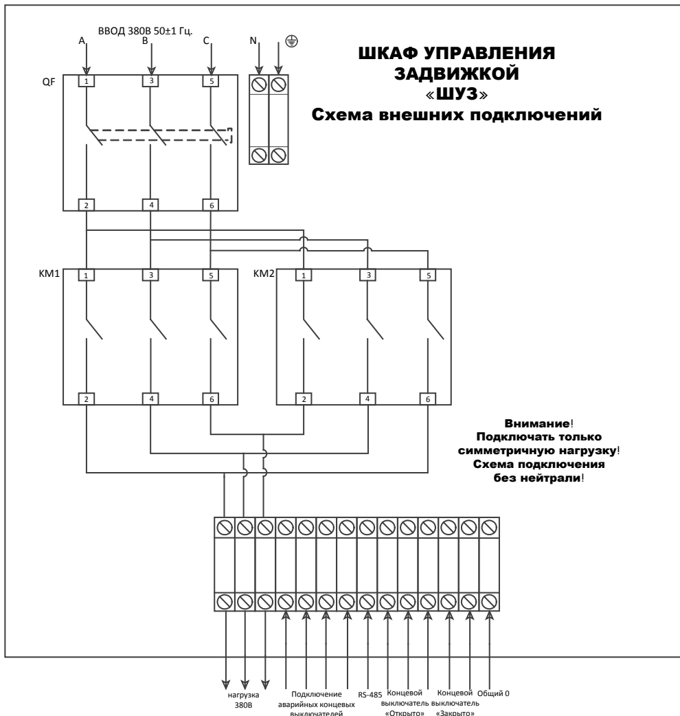
Рисунок 2-а. Схема внешних подключений к шкафу при 380В.
