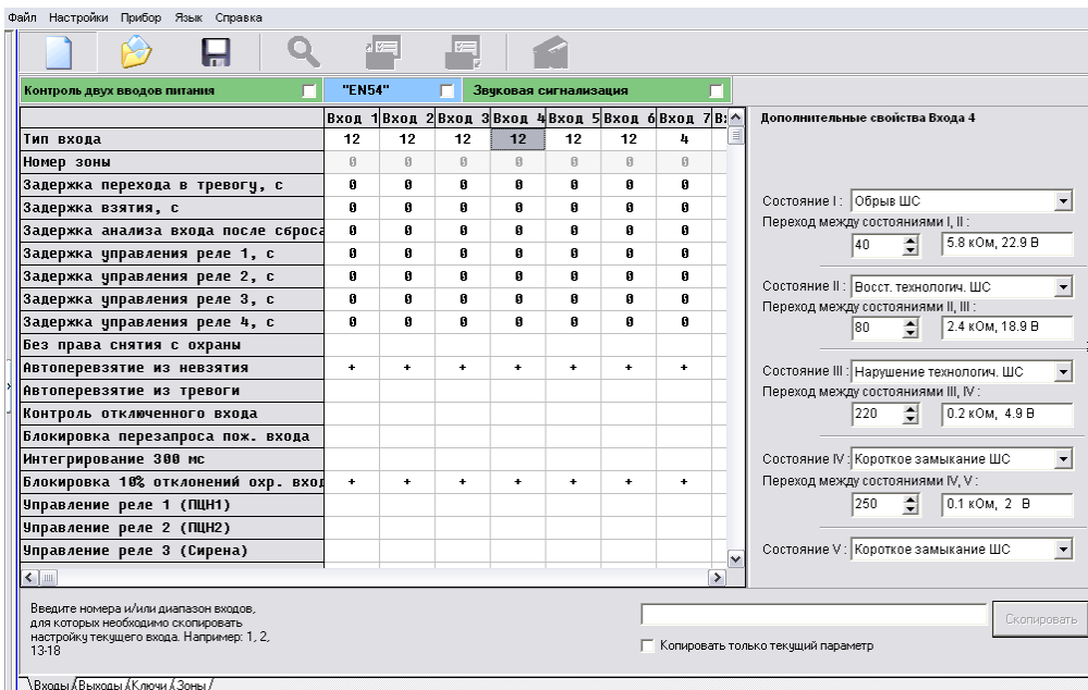
Рисунок 6. Входы «Закрытие», «Открытие».
