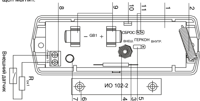
Рисунок 1 «Ладога МК-РК» исполнение 3
