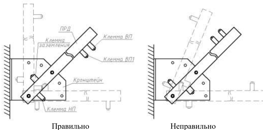
Рисунок 2.6 Установка ПРД
