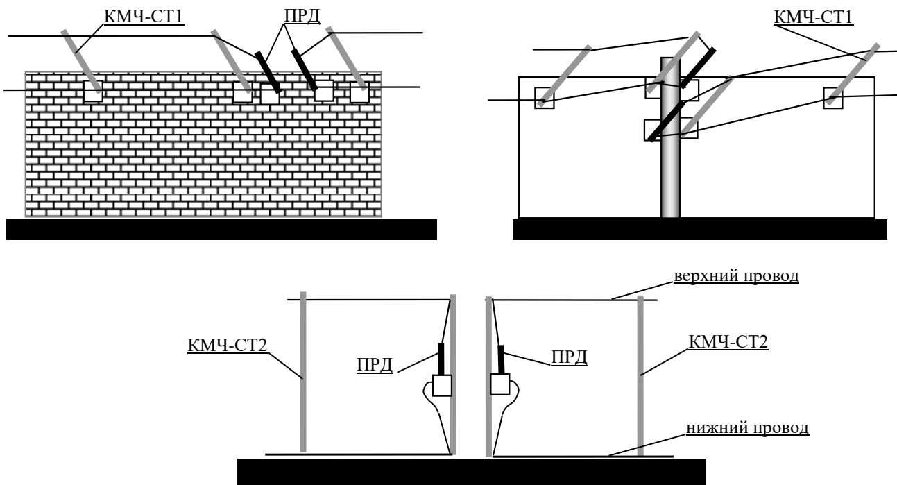
Рисунок 1.2 Расположение блоков ПРД смежных участков охраны относительно друг друга на ограждении и при приземном варианте установки извещателя
