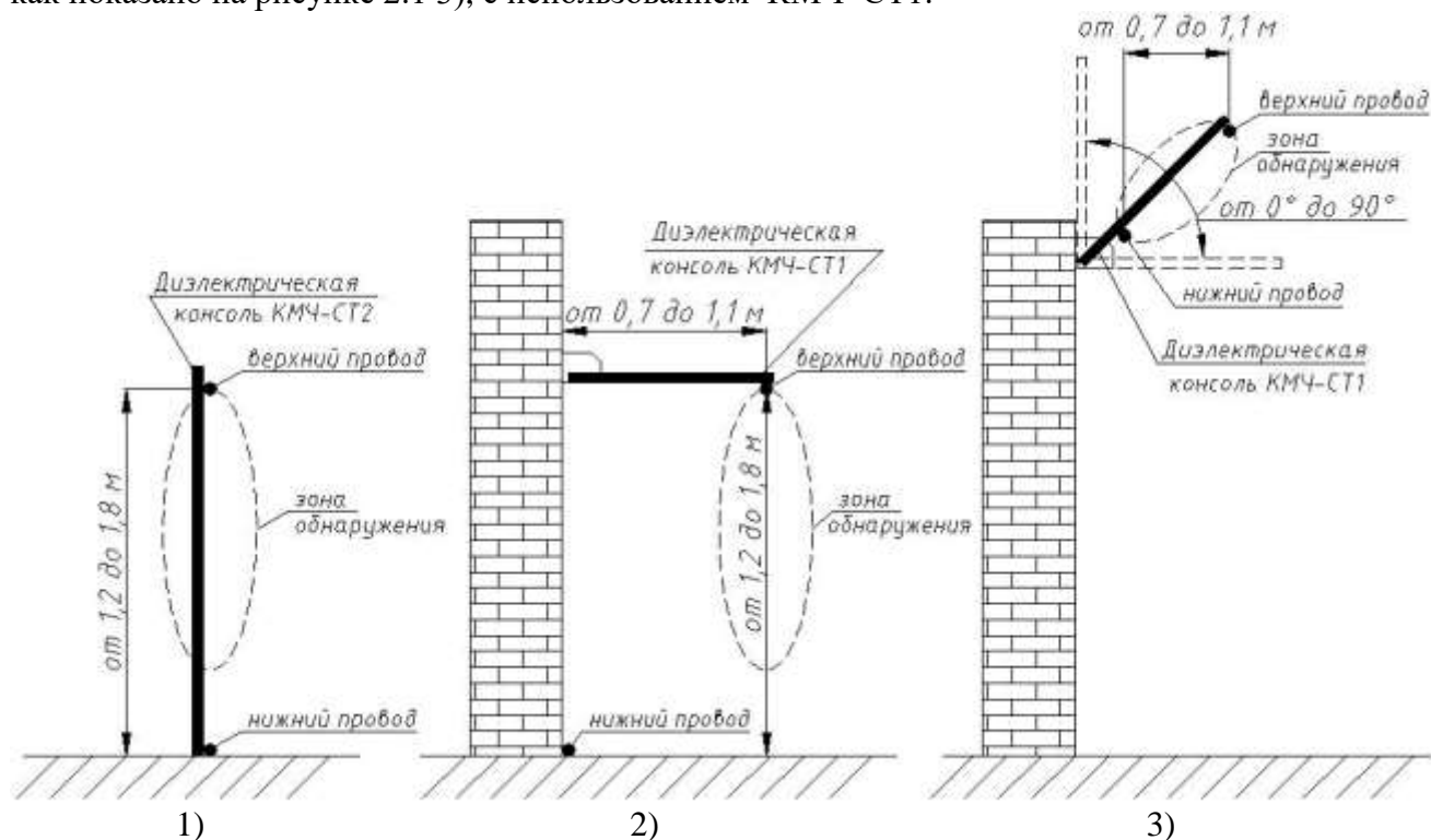
Рисунок 2.1 Варианты размещения линейной части извещателя
