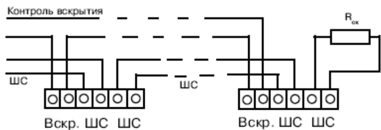
а) параллельно оконечному элементу (режим КЗ)
