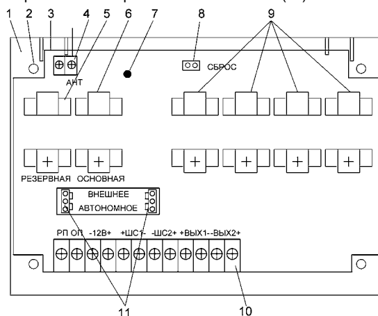
Рисунок 1 – БКВ-РК со снятой крышкой
