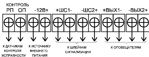
Рисунок 2 – Клеммная колодка для подключения внешних элементов
