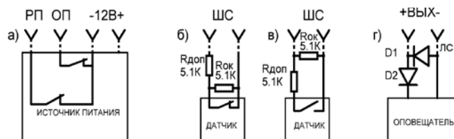
Рисунок 3 – Схемы подключения внешних устройств
