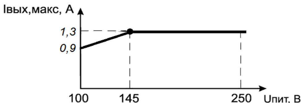
Рис. 1. Зависимость максимального выходного тока I_{\text{вых, макс}} от напряжения питания сети U_{\text{пит}}
