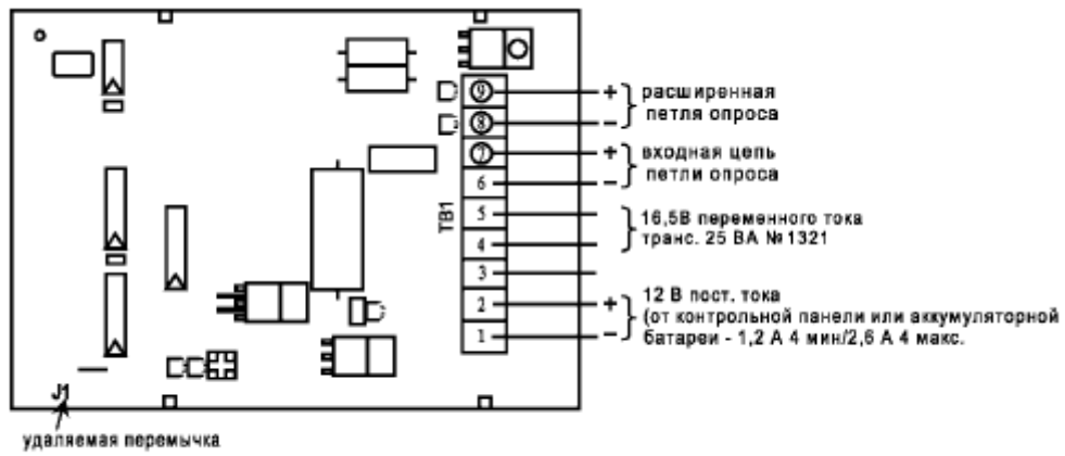
Рисунок 1 – Проводные соединения
