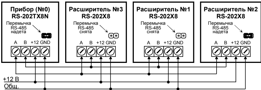
Рис. 11. Пример подключения расширителей к прибору.
