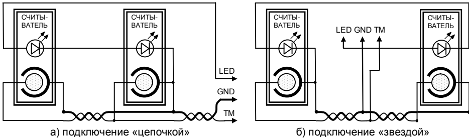
Рис. 9. Подключение двух считывателей
