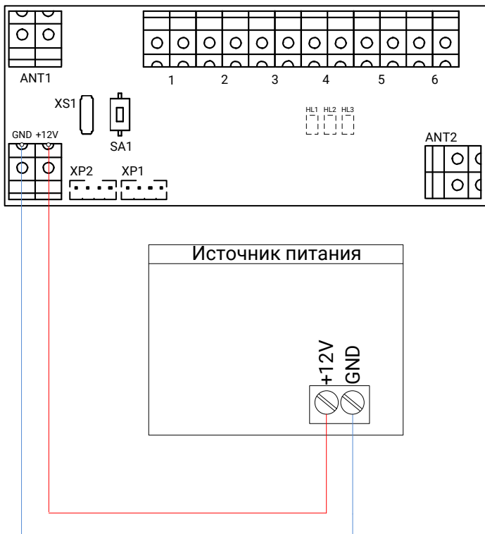
Рисунок 3. Схема подключения внешнего источника питания
