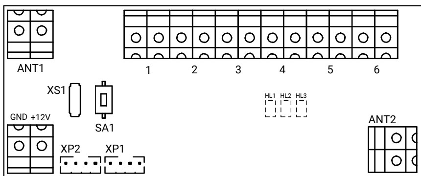
Рисунок 1. Плата приёмника
