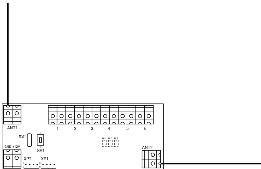
Рисунок 4. Схема подключения антенн
