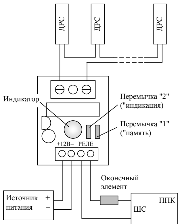
Схема подключения
