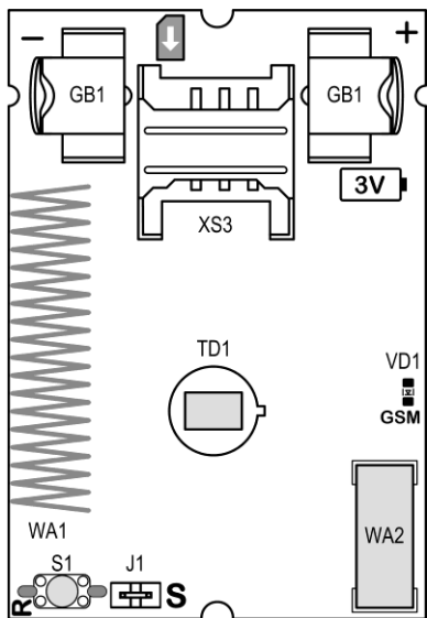
Рис.2 Плата сигнализатора
