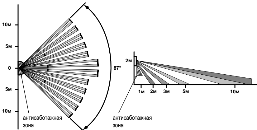
Рис.11 Диаграмма зоны обнаружения
