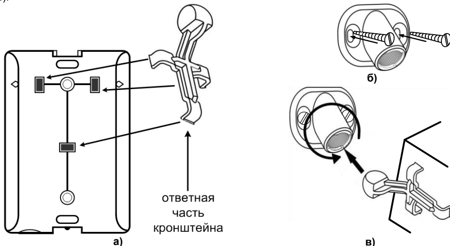
Рис.13 Установка кронштейна и сигнализатора
