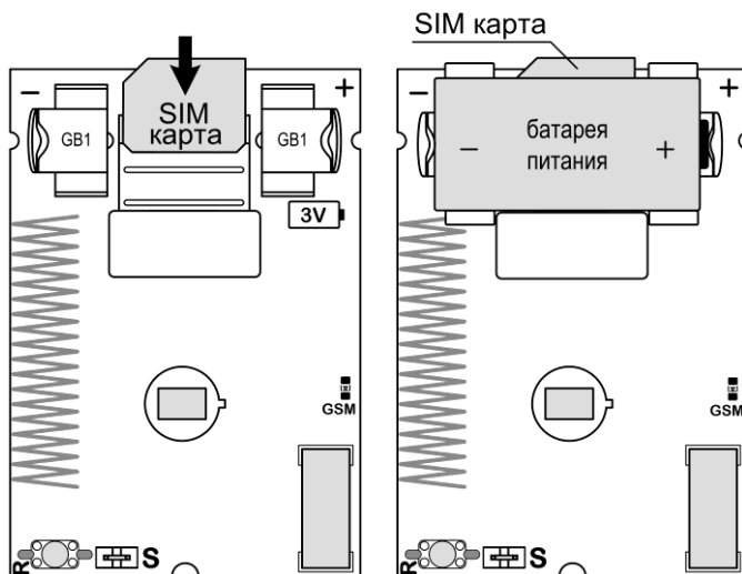
Рис.9 Установка SIM карты. Установка батареи питания
