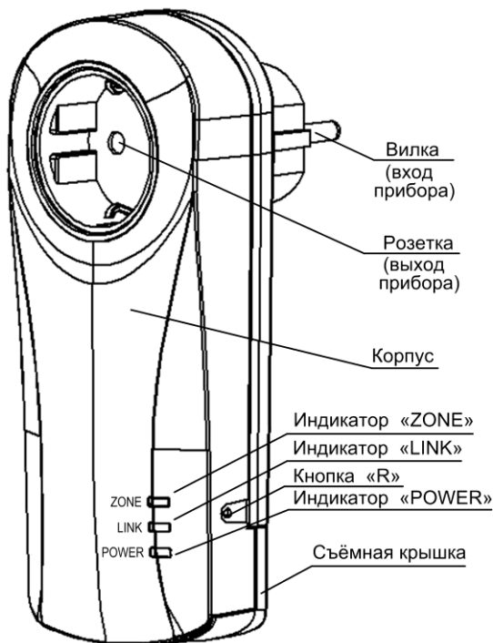
Рис.1 Внешний вид GSM розетки
