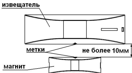
Рис. 11 Общий вид извещателя
