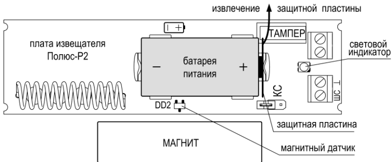
Рис.10 Плата извещателя Полюс-Р2
