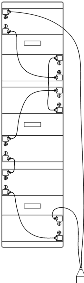
Рисунок 11 — схема соединений АКБ
