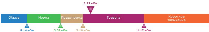
Рисунок 25. Шкала порогов пожарного шлейфа
