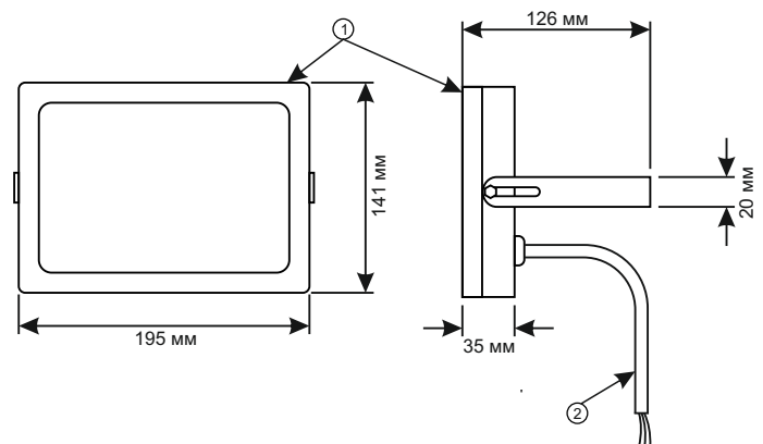
Рисунок 1 — Общий вид изделия
