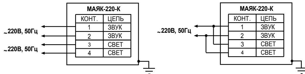
Рис.1. Схема подключения.
